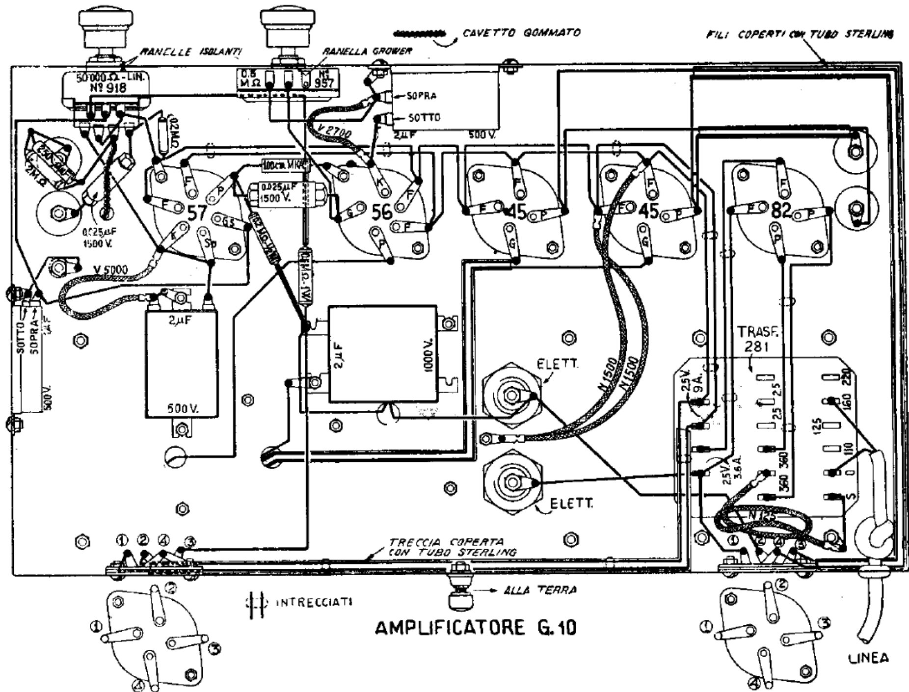
Schema costruttivo dell'amplificatore G. 10.
